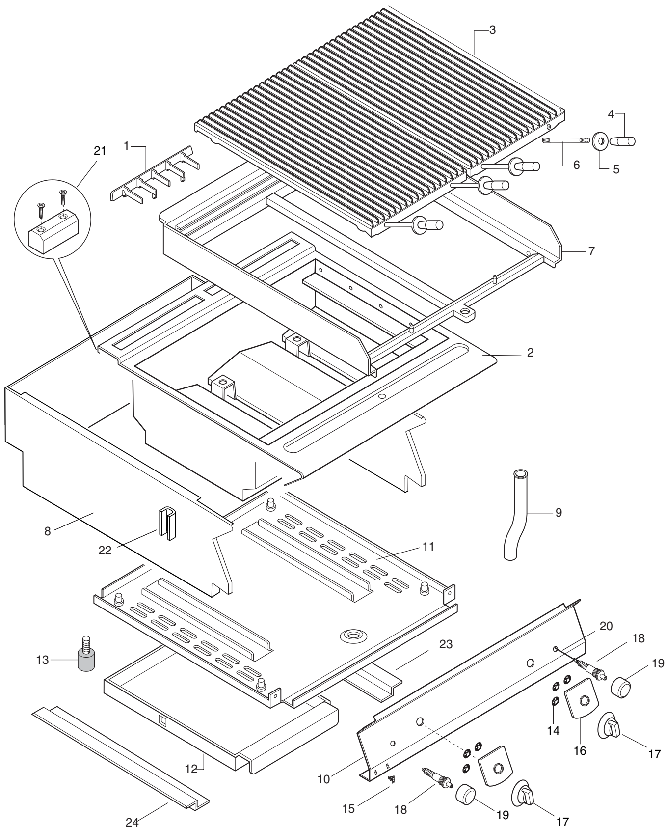
GRIGLIA GAS PIETRA LAVICA TOP N700 GAS LAVA STONE GRILL TOP N700
